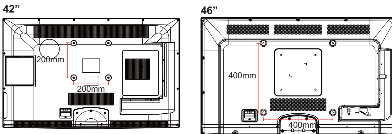
Dimensiones para el Patrón de agujeros de montaje
