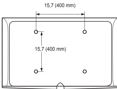
VUE ARRIÈRE
