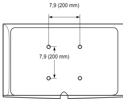
VUE ARRIÈRE
