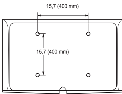
VUE ARRIÈRE
