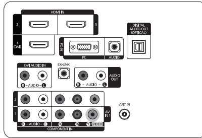
DÉTAIL DU PANNEAU DES PRISES 5,2" H X 6,6" W
