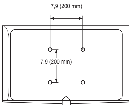
VUE ARRIÈRE
